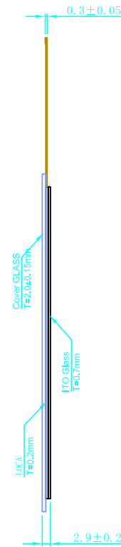
侧视图
