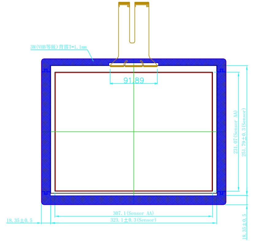
背视图
